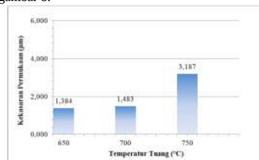
Gambar 8. Grafik Data Pengujian Kekasaran Permukaan Terhadap Temperatur Tuang pada Ukuran Butir Lempung 100 Mesh.
