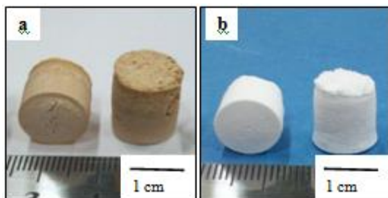
Gambar 1. (a) Green Bodies dan (b) Sintered Bodies Sampel pada Penambahan Jumlah TCP 9 Gram dan Kecepatan Pengadukan 100 rpm
