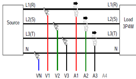
Gambar 2. Konfigurasi Pemasangan alat ukur
