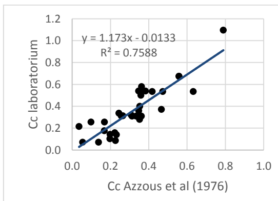
Gambar 10. Perbandingan Nilai Cc Laboratorium dan Hasil Rumus Azzouz et al. (1976)
