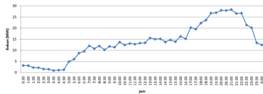
Gambar 3 Grafik estimasi pola beban dasar televisi seluruh rumah tangga di pekanbaru
