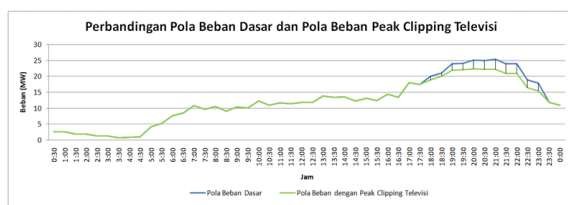
Gambar 4 Perubahan pola beban dengan peak clipping televisi rumah tangga di Pekanbaru
