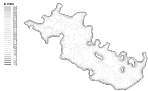
Gambar 3. Kontur dasar Waduk Sei Paku tahun 2014
