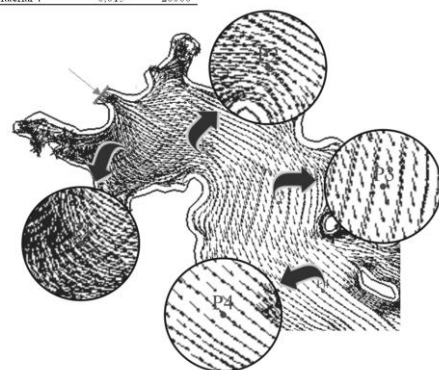
Gambar 4. Hasil kalibrasi arah dan kecepatan aliran yang sesuai dengan kondisi lapangan
