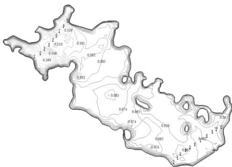
Gambar 12. Perubahan dasar waduk ( bed change ) pada kala ulang 5 tahun selama 2160 jam (3 bulan)
