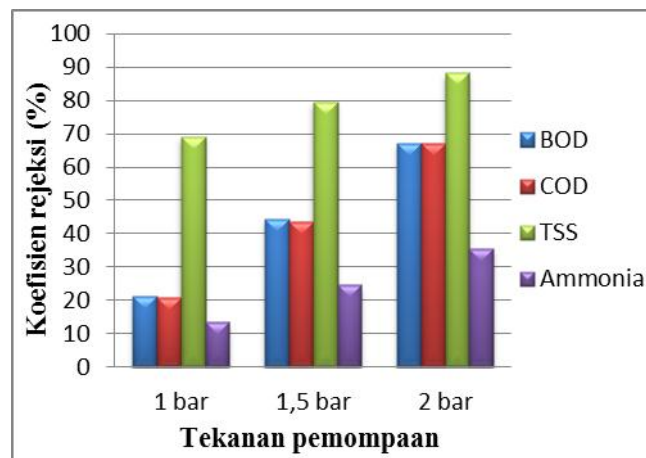
Gambar 3.2 Pengaruh tekanan pemompaan membran ultrafiltrasi terhadap penyisihan BOD, COD, TSS dan ammonia
