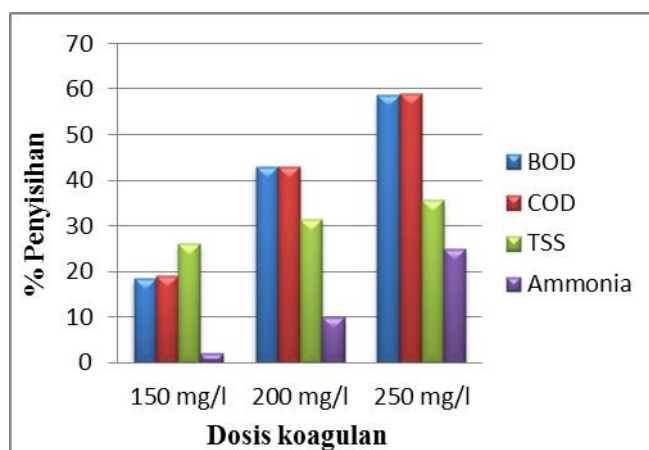
Gambar 3.1 Efektifitas proses koagulasi
