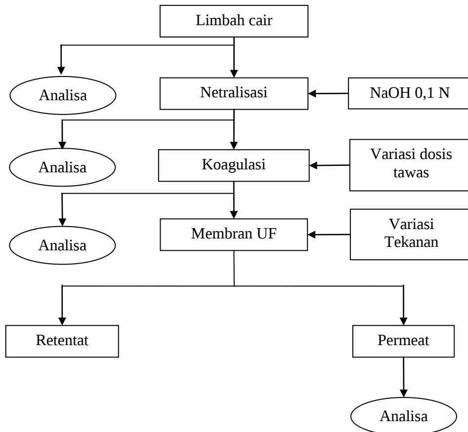
Gambar 2.1 Skema proses pengolahan limbah cair industri karet
