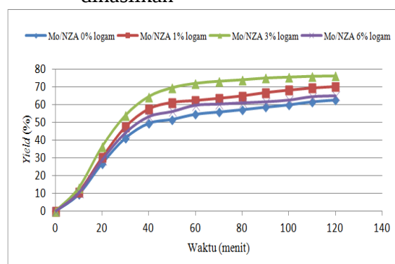
Gambar 3. Pengaruh variasi persentase pengembunan logam Mo/NZA dengan rasio katalis 9% terhadap biomassa pada yield bio-oil yang dihasilkan
