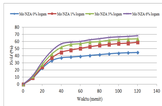
Gambar 2. Pengaruh variasi persentase pengembunan logam Mo/NZA dengan rasio katalis 6% terhadap biomassa pada yield bio-oil yang dihasilkan
