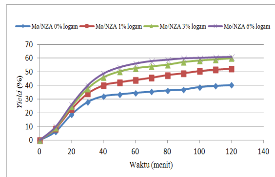
Gambar 1. Pengaruh persentase pengembunan logam pada rasio katalis 3% terhadap biomassa pada yield bio-oil yang dihasilkan
