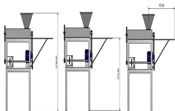
Gambar 2.3 Dimensi Akhir
