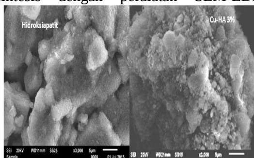
Gambar 1. Perbandingan Foto SEM HAp Hasil Sintesis dengan Katalis Cu-HAp
