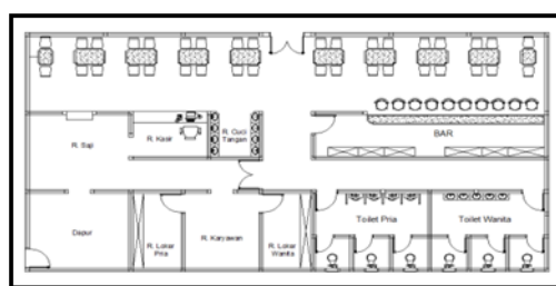
Gambar 4.13 Denah Bangunan Restoran Sumber: Hasil Pengembangan Desain (2015)
