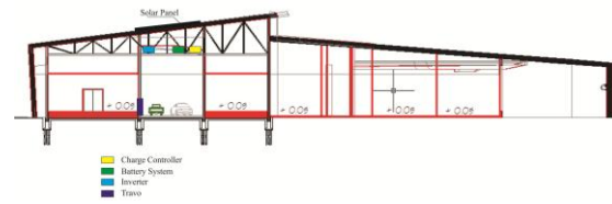
Gambar 14. Potongan Skematik Utilitas Photovoltaic
