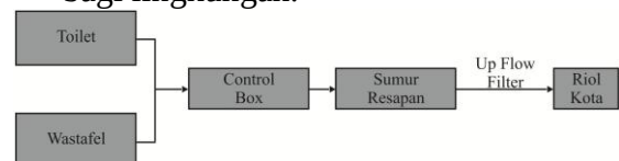
Gambar 11. Skema Gray Water Sumber: Hasil Pengembangan Desain (2015)
