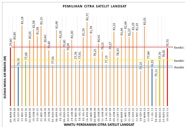
Gambar 4.1 Grafik Pemilihan Data Citra Satelit Landsat
