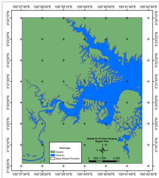
Gambar 4.12 Hasil klasifikasi Daratan dan Perairan Pada Kondisi 3 (Perekaman Tanggal 18 Desember 2013)
