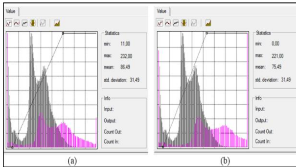
Gambar 4.4 Penyesuaian Histogram Band 5 Citra Landsat-7 ETM+ Perekaman Tanggal 01 September 2000 Sebelum Dikoreksi Radiometrik (a) dan Setelah Dikoreksi Radiometrik (b)
