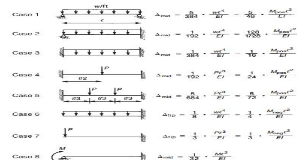
Gambar 2 Perhitungan Defleksi Metode Westergrand (Sumber: MacGreor dkk, 2012)
