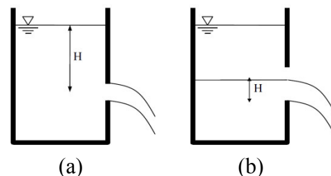
Gambar 1. Aliran melalui lubang (a) dan peluap (b)
