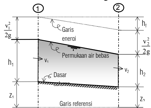
Gambar 4. Energi dalam aliran saluran terbuka
