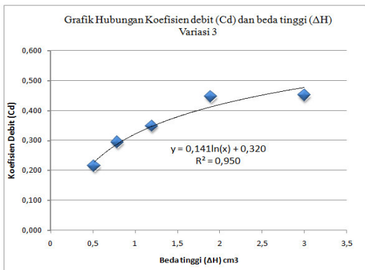
Gambar 11. Grafik Regresi Logarithmic variasi 3
