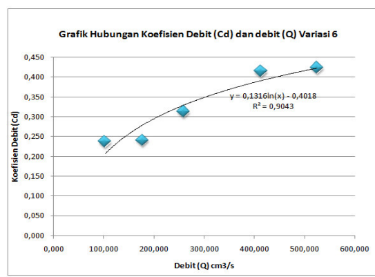
Gambar 18. Grafik Regresi Logarithmic variasi 6
