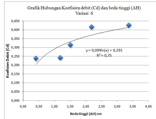
Gambar 13 Grafik Regresi Logarithmic variasi 6
