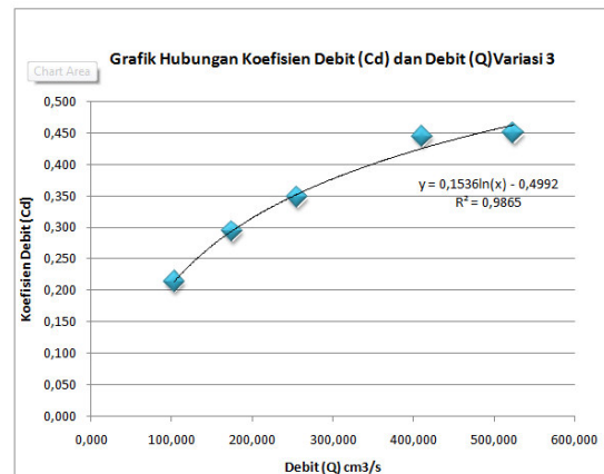
Gambar 16. Grafik Regresi Logarithmic variasi 3
