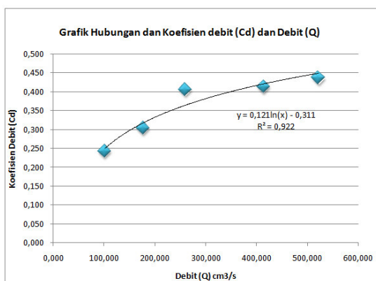
Gambar 14. Grafik Regresi Logarithmic variasi 1
