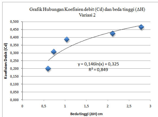
Gambar 10. Grafik Regresi Logarithmic variasi 2
