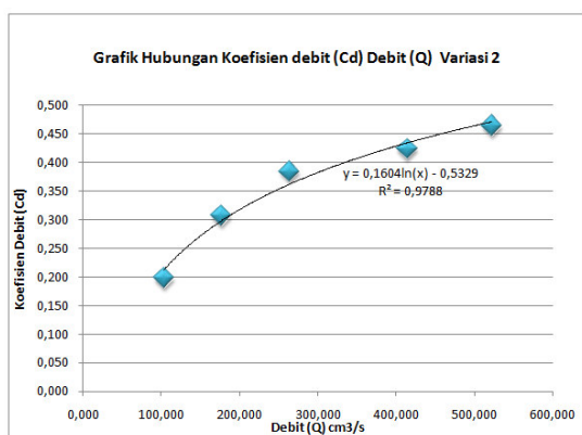
Gambar 15. Grafik Regresi Logarithmic variasi 2
