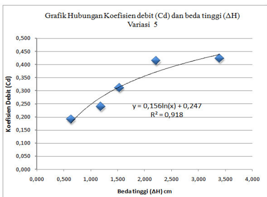
Gambar 12. Grafik Regresi Logarithmic variasi 5
