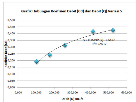
Gambar 17. Grafik Regresi Logarithmic variasi 5
