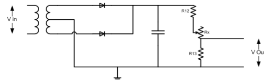
Gambar 2.7 Sensor tegangan
