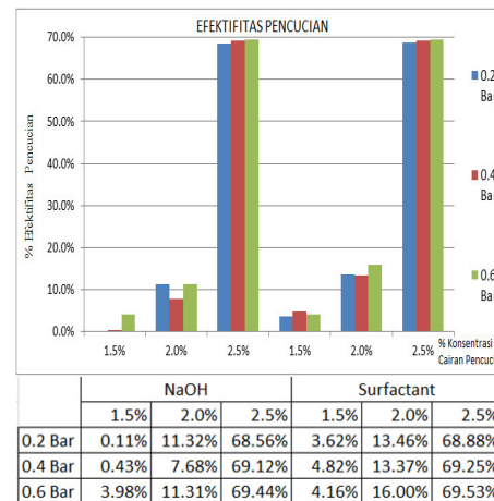
Gambar 3. Efektifitas Pencucian Berdasarkan Tekanan dan Konsentrasi Cairan Pencuci
