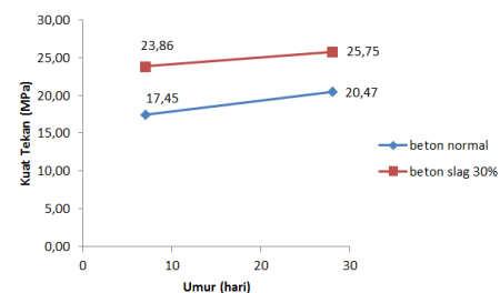
Gambar 6. Grafik kuat tekan beton
