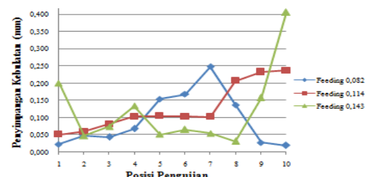
Gambar 4.3 Grafik Perbandingan Penyimpangan Kebulatan Berdasarkan Lingkaran Daerah Minimum
