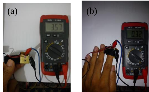
Gambar 3.1 pengujian sensor menggunakan multimeter digital
