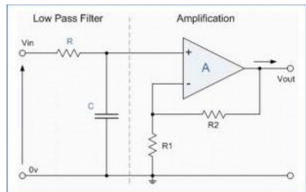
Gambar 1.6 Rangkaian LPF aktif (Purnama, Agus. 2015)
