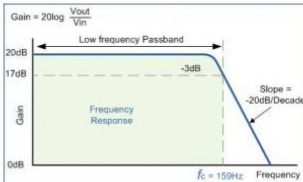
Gambar 1.8 Respon frekuensi LPF aktif (Purnama, Agus. 2015)
