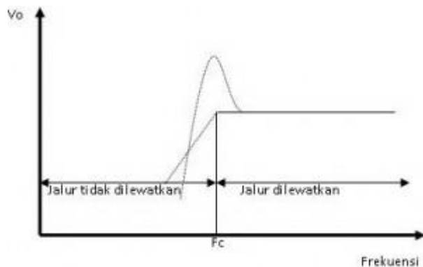
Gambar 1.5 Karakteristik HPF RC (Purnama, Agus. 2012)
