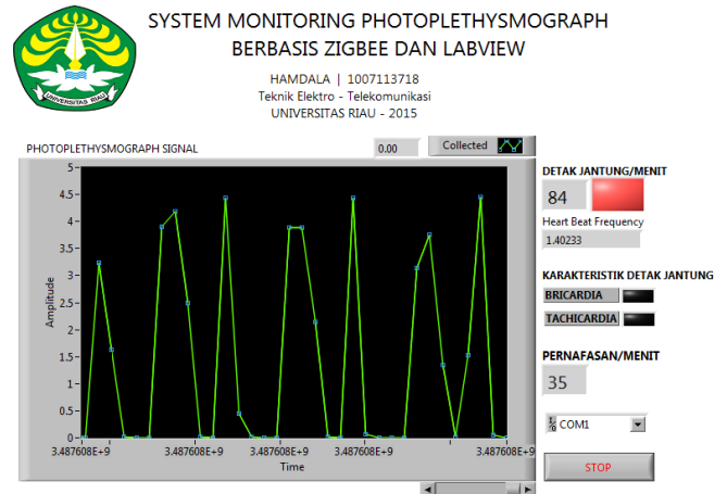
Gambar 3.5 Sistem monitoring PPG berbasis labview yang dibuat dengan serial interface
