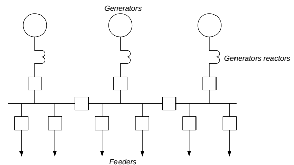
Gambar 2.1 Reaktor Generator (Skrotzki, 1954: 435)
