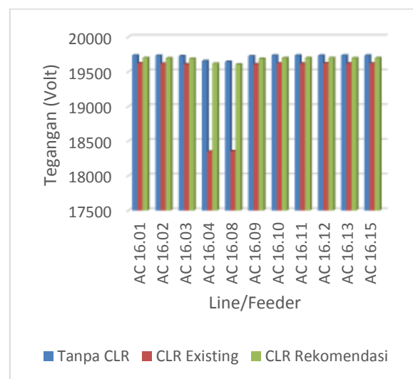
Gambar 4.10 Tegangan pada masing-masing feeder pada substation AC 16 per-studi kasus
