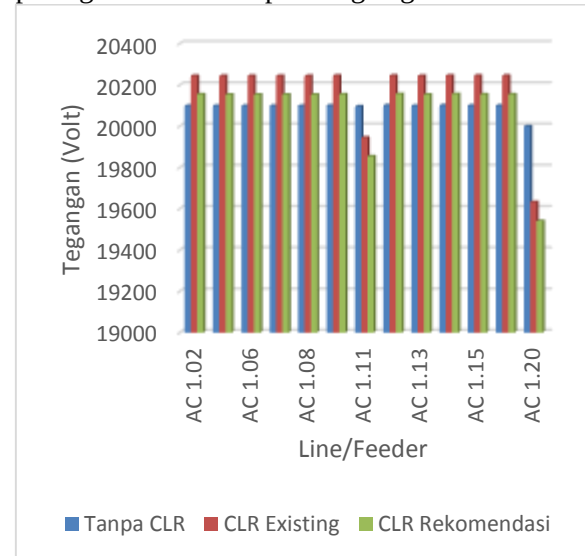
Gambar 4.2 Tegangan pada masing-masing feeder pada substation AC 1 per-studi kasus
