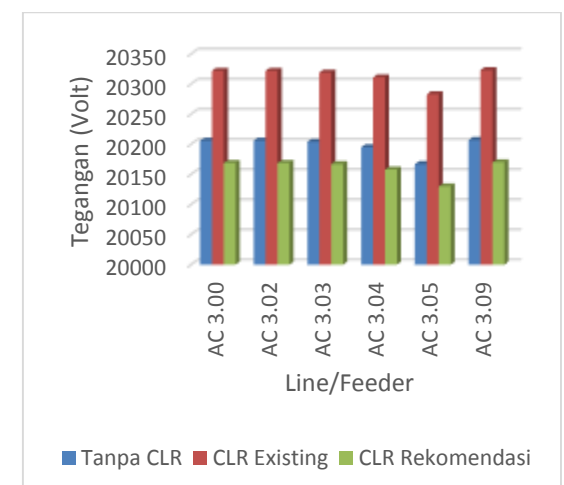
Gambar 4.4 Tegangan pada masing-masing feeder pada substation AC 3 per-studi kasus
