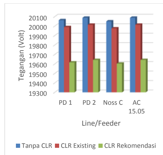
Gambar 4.9 Tegangan pada masing-masing feeder pada substation AC 15 per-studi kasus
