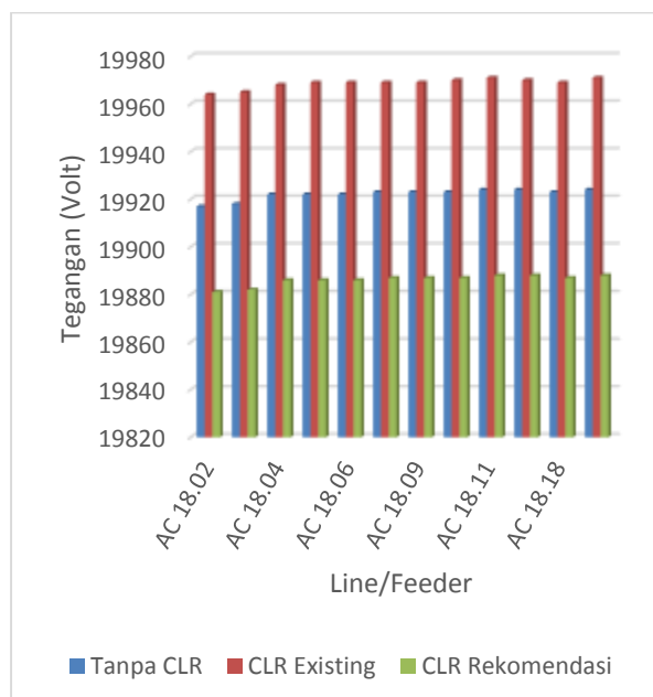
Gambar 4.12 Tegangan pada masing-masing feeder pada substation AC 18 per-studi kasus
