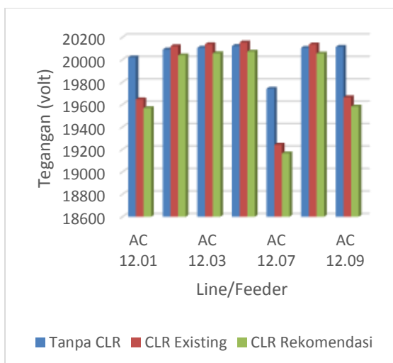
Gambar 4.7 Tegangan pada masing-masing feeder pada substation AC 12 per-studi kasus
