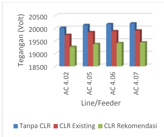
Gambar 4.5 Tegangan pada masing-masing feeder pada substation AC 4 per-studi kasus
