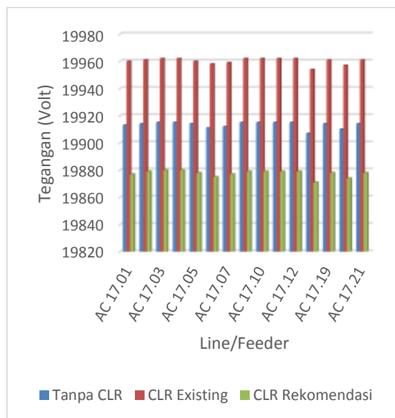
Gambar 4.11 Tegangan pada masing-masing feeder pada substation AC 17 per-studi kasus
