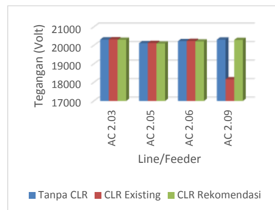
Gambar 4.3 Tegangan pada masing-masing feeder pada substation AC 2 per-studi kasus
