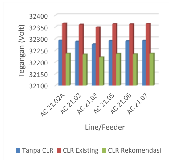
Gambar 4.13 Tegangan pada masing-masing feeder pada substation AC 21 per-studi kasus
