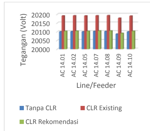
Gambar 4.8 Tegangan pada masing-masing feeder pada substation AC 14 perstudi kasus
