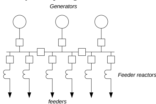
Gambar 2.5 Reaktor penyulang (Skrotzki, 1954: 435)
