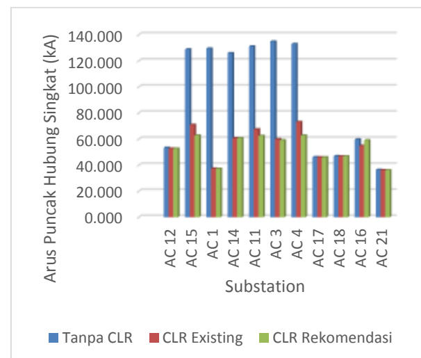
Gambar 4.1 Arus Puncak Hubung Singkat Pada Masing-masing Substation Perstudi-kasus
