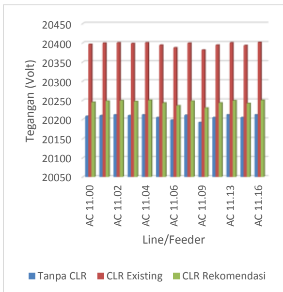
Gambar 4.6 Tegangan pada masing-masing feeder pada substation AC 11 per-studi kasus
