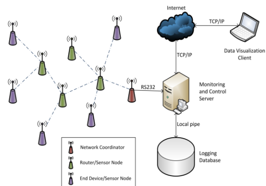
Gambar 2 Arsitektur WSN
