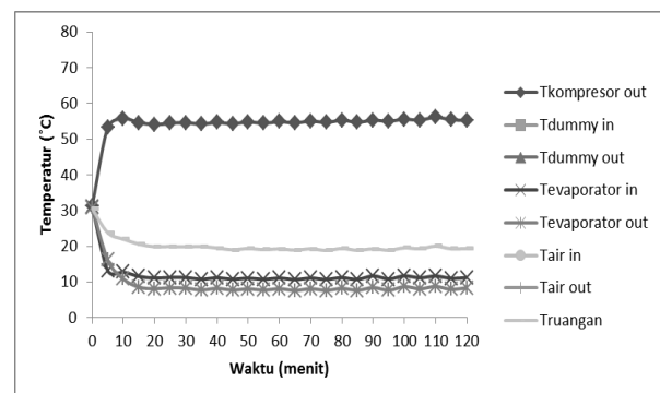
Gambar 6. Grafik Temperatur AC Standar dengan Beban Pendinginan 1000 W
