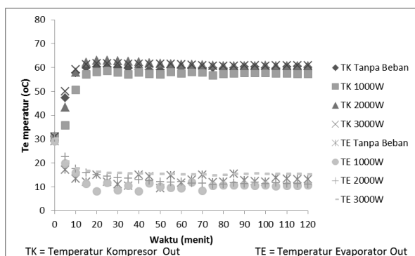
Gambar 14. Grafik Temperatur Kompresor ACWH pada Setiap Beban Pendinginan
