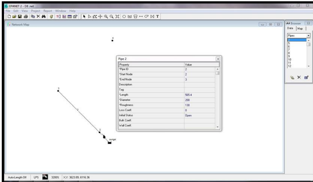
Gambar 3. Memberikan Nomor pada node-node (simpul pipa)
