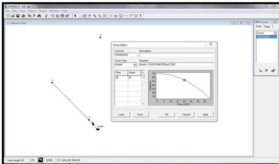
Gambar 4. Input Debit dan Head pada Pompa
