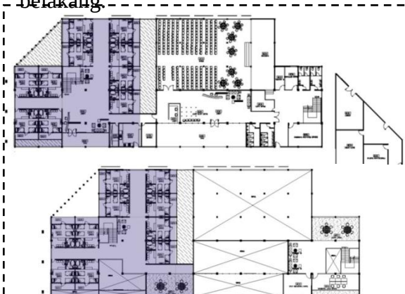
Gambar 3.10. Denah Pendukung Satu
