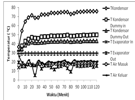
Gambar 4. Grafik Temperatur Standar
