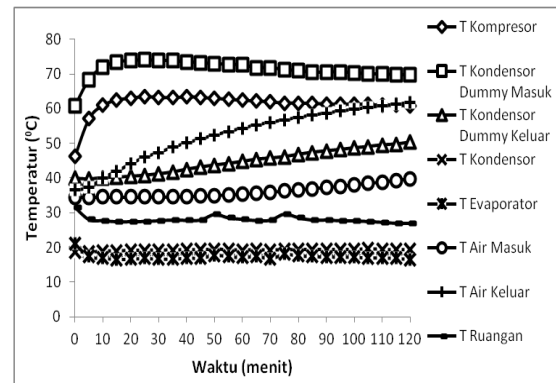
Gambar 11. Grafik Temperatur Dengan Penambahan Kondensor Dummy Beban 3000 W
