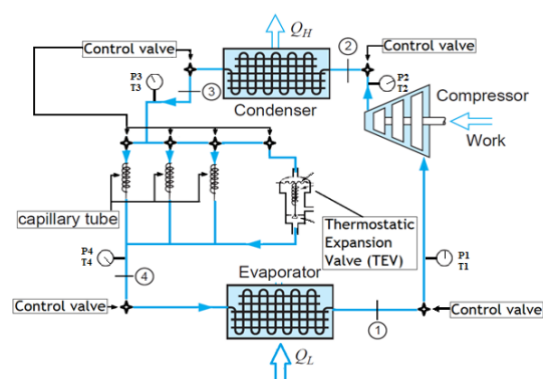
Gambar 6 Diagram Skematik Fasilitas Pengujian Mesin Pendingin [5]
