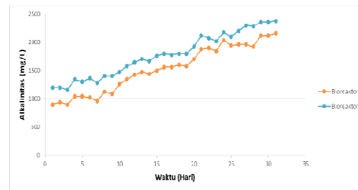
Gambar 3. Perubahan Alkalinitas Selama Transien
