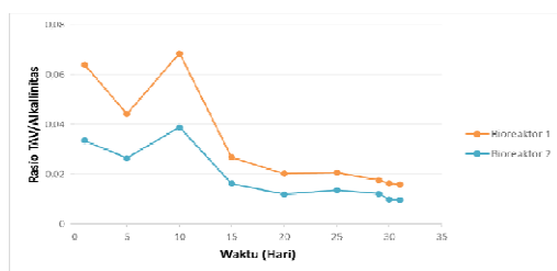
Gambar 6. Kestabilan Bioreaktor pada Kondisi Start-Up
