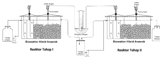
Gambar 1. Rangkaian Peralatan Pengolahan dengan Menggunakan Bioreaktor Hibrid Anaerob Dua Tahap Bermedia Batu
