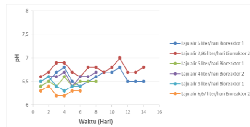
Gambar 7. Hubungan antara Laju Alir terhadap pH pada Proses Kontinu
