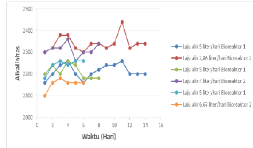
Gambar 8. Hubungan antara Laju alir terhadap Alkalinitas pada Proses Kontinu
