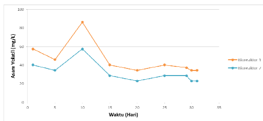
Gambar 5. Perubahan Asam Volatil Selama Transien
