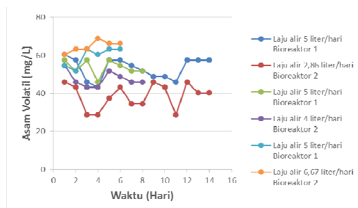
Gambar 9. Hubungan antara Laju alir terhadap Asam Volatil pada Proses Kontinu
