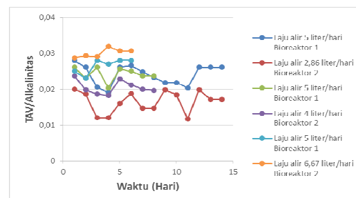
Gambar 10. Kestabilan Bioreaktor Selama Proses Kontinu
