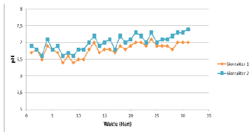
Gambar 2. Perubahan pH Selama Transien
