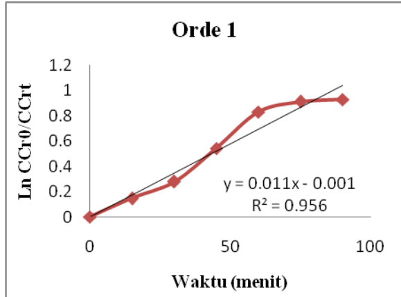
Gambar 4.3 Model Kinetika Orde Satu Untuk Variasi Waktu Kontak
