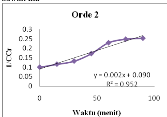
Gambar 4.4 Model Kinetika Orde Dua Untuk Variasi Waktu Kontak
