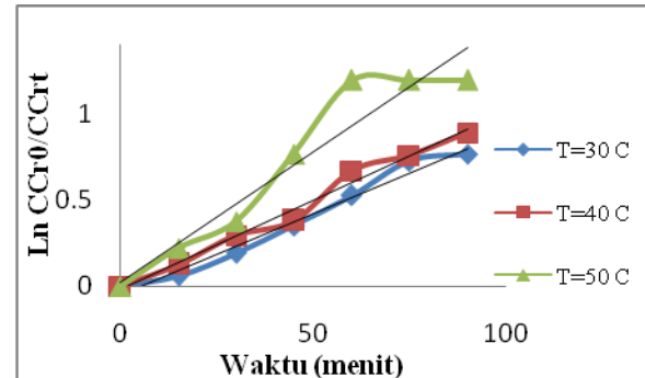
Gambar 4.5 Pengaruh Temperatur Terhadap Laju Adsorpsi
