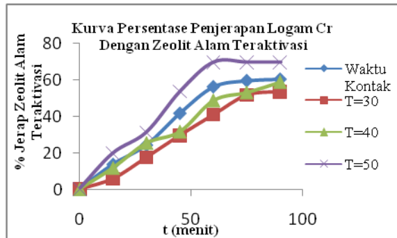
Gambar 4.1 Pengaruh Waktu (t) Terhadap Efisiensi Penjerapan (%) Logam Cr oleh Zeolit Alam Teraktifasi
