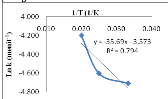
Gambar 4.6 Hubungan antara \ln k (Menit -1 ) terhadap 1/T
