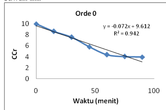
Gambar 4.2 Model Kinetika Orde Nol Untuk Variasi Waktu Kontak
