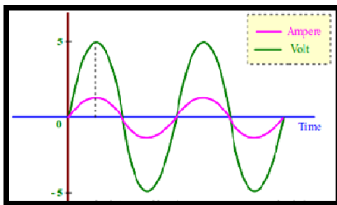
Gambar 2. Bentuk gelombang beban resistif
