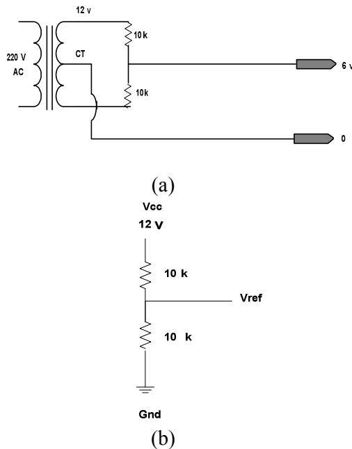
Gambar 8. (a) Sensor Tegangan (b) Rangkaian Pembagi Tegangan
