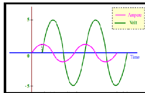
Gambar 6. Beban Kapasitif
