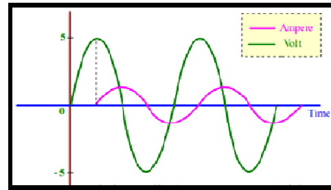
Gambar 4. Bentuk Gelombang Beban Induktif
