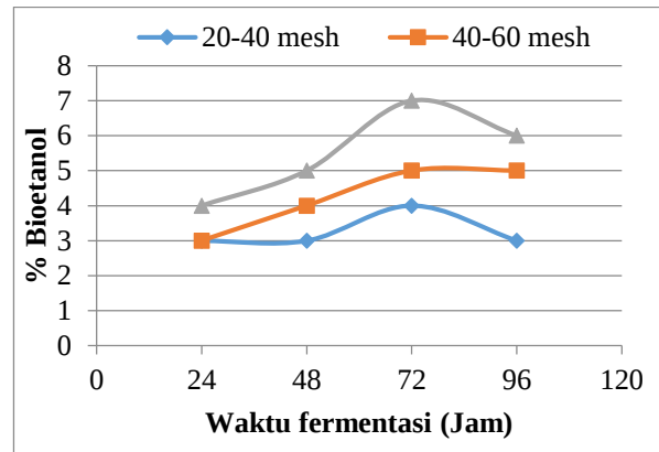
Gambar 3.1 Hasil Konsentrasi Bioetanol pada proses SFS dengan variasi ukuran partikel
