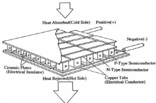
Gambar 1 Kontruksi Thermoelektrik [6]
