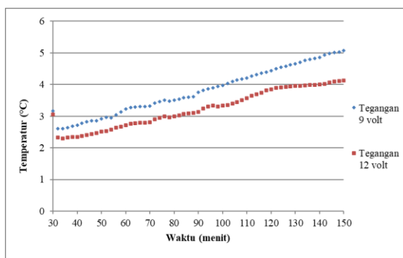
Gambar 5 Grafik Perbandingan Temperatur Darah Dengan Variasi Input Tegangan 9 volt dan 12 volt
