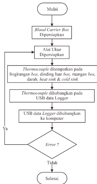
Gambar 3 Diagram Alir Instalasi Alat Ukur
