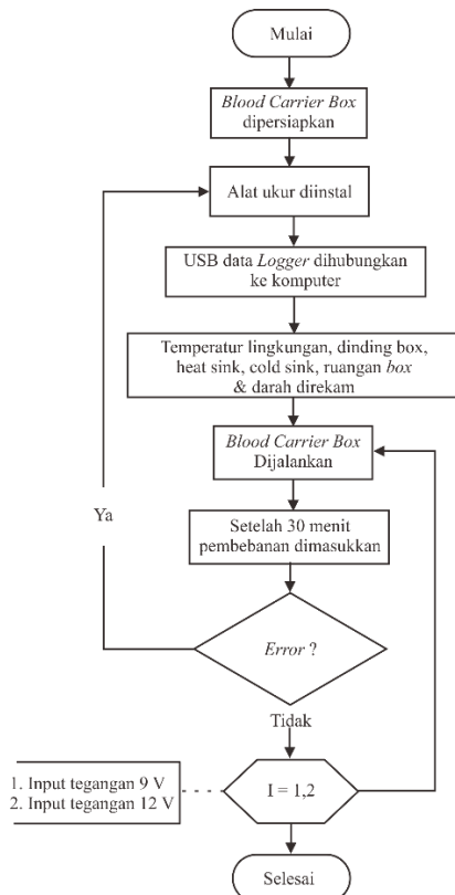
Gambar 4 Diagram Alir Pengambilan Data
