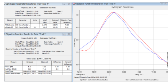
Gambar 4 Hasil Kalibrasi Metode Clark Durasi 6 jam
