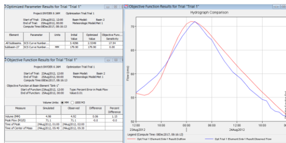
Gambar 3 Hasil Kalibrasi Metode Snyder Durasi 6 jam
