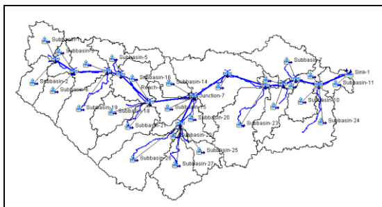
Gambar 2. Konfigurasi DAS Siak Bagian Hulu dalam Basin Model HEC-HMS
