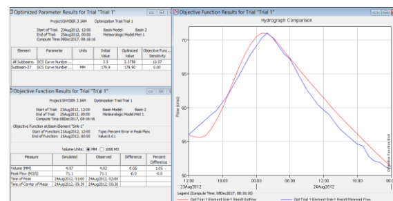
Gambar 5 Hasil Kalibrasi Metode Snyder Durasi 3 jam
