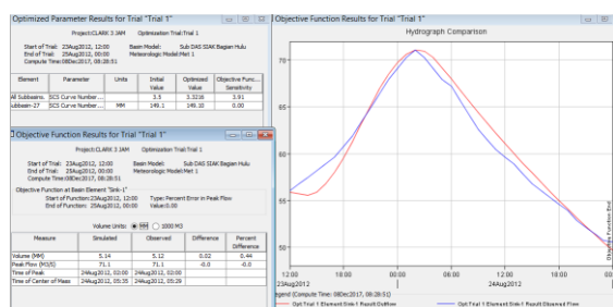
Gambar 3 Hasil Kalibrasi Metode Clark Durasi 3 jam
