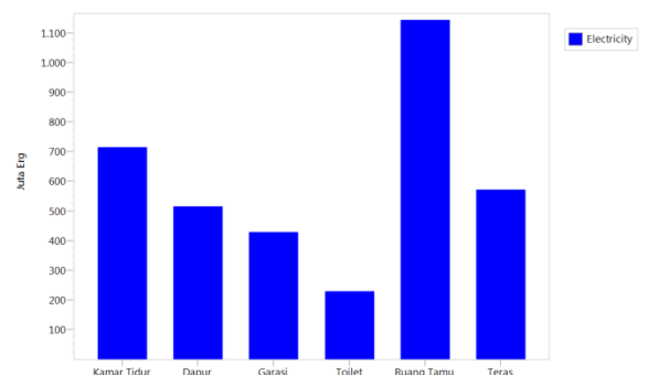
Gambar 6. Grafik Sebelum Konservasi Daya Terpasang 1300 VA
