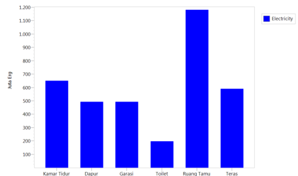
Gambar 6. Grafik Sebelum Konservasi Daya Terpasang 1300 VA
