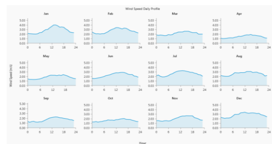
Gambar 4.2 Kurva rata-rata kecepatan angin selama setahun Di Pekanbaru
