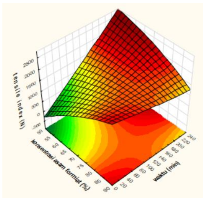
Gambar 5. Pengaruh Konsentrasi Asam Formiat dan Waktu Reaksi terhadap Kuat Tarik Pulp Pada Nisbah Cairan-Padatan 20/1
