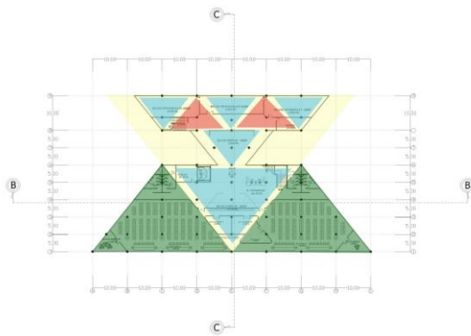
Gambar 7 Denah lantai pada bangunan Perpustakaan dan Kearsipan
