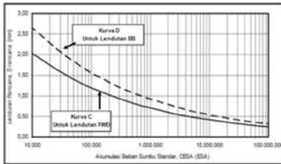
Gambar 1. Hubungan antara lendutan rencana dari lalu lintas (Bina Marga, 2005)
