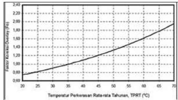
Gambar 3. Faktor koreksi tebal lapis tambah ( overlay ) ( F_o )
