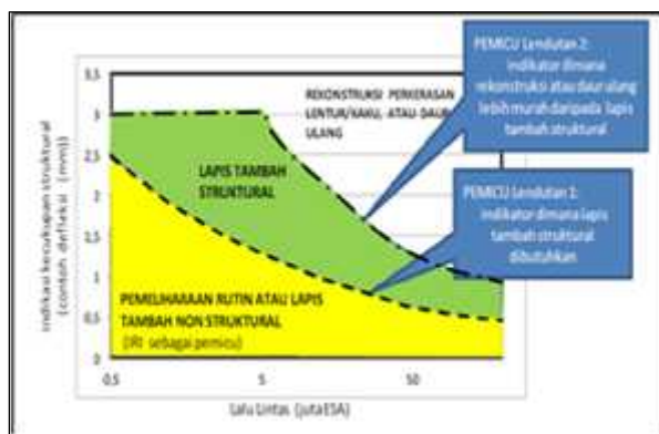
Gambar 4. Pemicu konseptual untuk penanganan pekerasan
