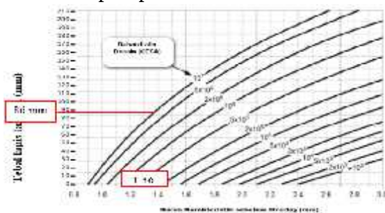
Gambar 11. Solusi overlay berdasarkan lendutan Benkelman Beam untuk WMAPT 41^\circ\text{C}
