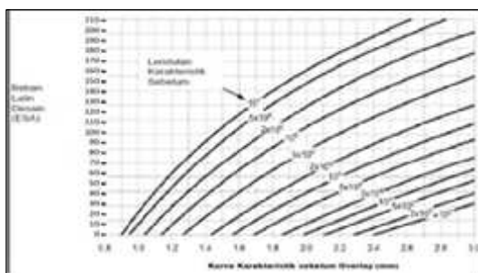
Gambar 6. Solusi overlay berdasarkan lendutan Benkelman Beam untuk WMAPI 41°C
