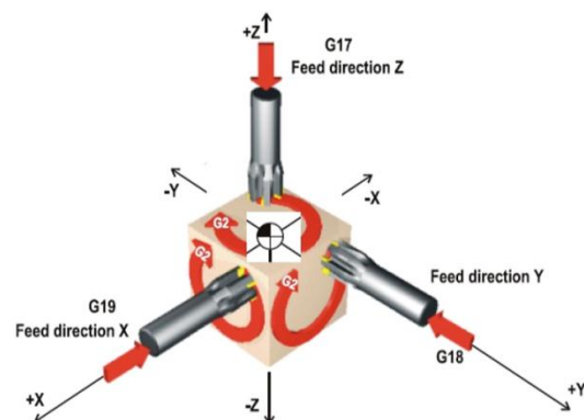
Gambar 3 Bidang Interpolasi Benda Kerja [7]
