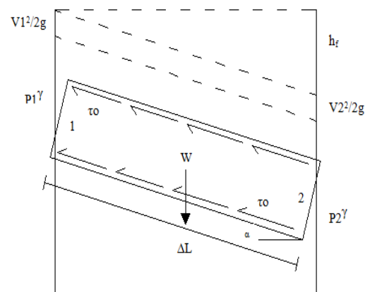
Gambar 2: Kehilangan tenaga pada aliran dalam pipa (sumber: Bambang triadmojo)
