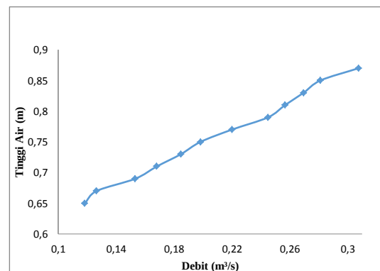
Gambar 4. Grafik Hubungan Antara Tinggi Air dengan Debit
