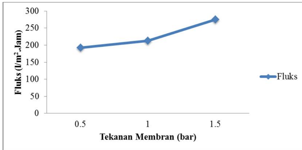
Gambar 3.3 Pengaruh Tekanan Pemompaan Terhadap Fluks Membran Ultrafiltrasi
