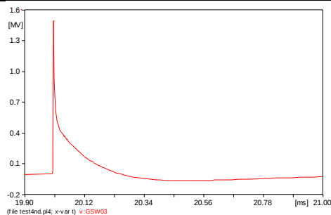
Gambar 6. tegangan impulse petir pada GSW mencapai puncaknya 1.4 Mega Volt.
