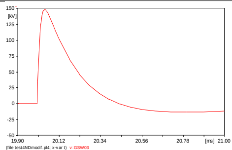
Gambar 9. tegangan impulse petir pada GSW mencapai puncaknya 150KV
