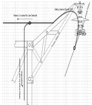
Gambar 1. Modifikasi GSW dengan penambahan isolator dan penambahan pentanahan sendiri.
