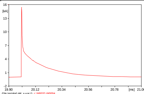
Gambar 7. Arus impuls petir pada Pentanahan terukur sebesar 15.5A.
