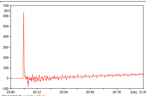
Gambar 8. Tegangan impuls petir pada Line A sebesar besar 600 kV.
