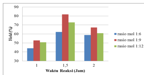
Gambar 1 Grafik Hubungan Antara Yield Biodiesel terhadap Waktu Reaksi Pada Kadar Logam Impregnasi 0%
