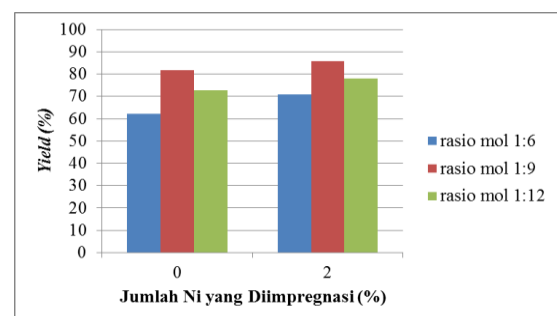
Gambar 3 Grafik Hubungan Antara Yield Biodiesel terhadap Jumlah Ni yang Diimpregnasi (%)
