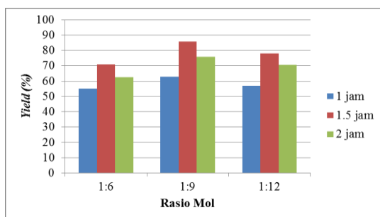
Gambar 2 Grafik Hubungan Antara Yield Biodiesel terhadap Rasio Mol Pada Kadar Logam Impregnasi 2%
