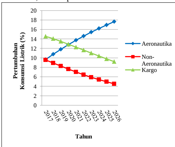
Gambar 4.2 Persentase Pertumbuhan Prakiraan Konsumsi Energi Listrik Per-Segmen Jasa Tahun 2017-2027
