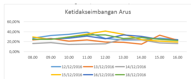
Gambar 6. Grafik pengukuran persentase (%) ketidakseimbangan arus pada siang hari (data diolah 2016)
