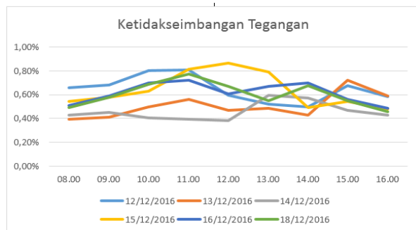
Gambar 8. Grafik pengukuran persentase (%) ketidakseimbangan tegangan pada siang hari (data diolah 2016)
