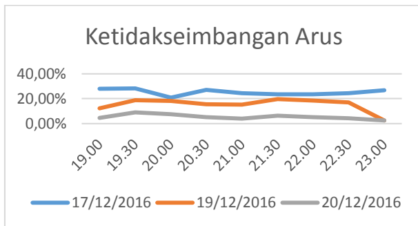
Gambar 7. Grafik pengukuran persentase (%) ketidakseimbangan arus pada malam hari (data diolah 2016)
