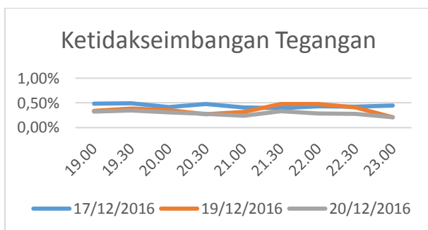
Gambar 9. Grafik pengukuran persentase (%) ketidakseimbangan tegangan pada malam hari (data diolah 2016)
