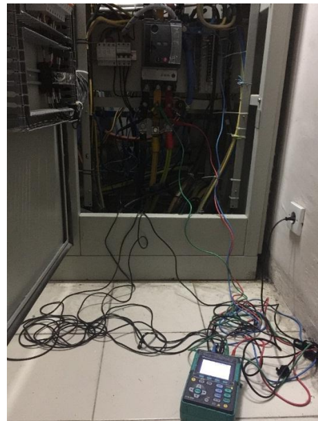
Gambar 1. Pengukuran Kualitas listrik pada Panel Utama Rumah Sakit Universitas Riau
