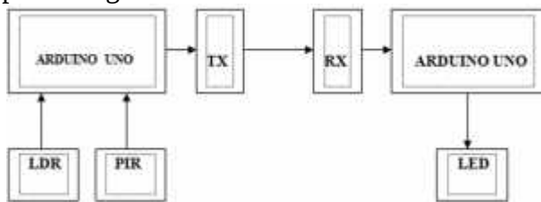
Gambar 3.6 Blok diagram Perancangan Sistem
