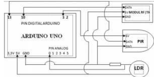
Gambar 3.7 Desain Rangkaian Transmitter
