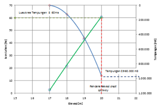
Gambar 6. Lengkung Kapasitas
