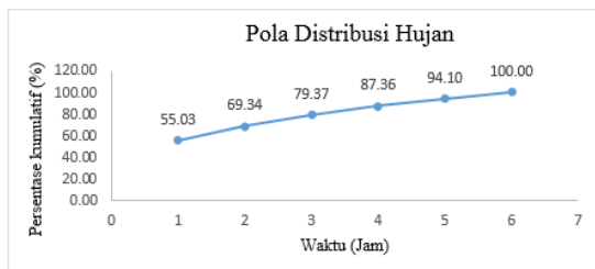
Gambar 2. Pola Distribusi Hujan
