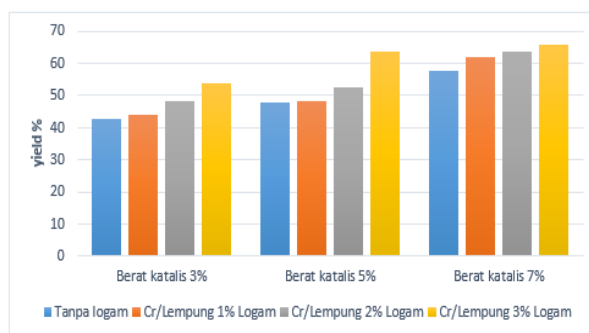
Gambar 2. Pengaruh Variasi Berat Katalis Cr/Lempung terhadap Yield Bio-Oil
