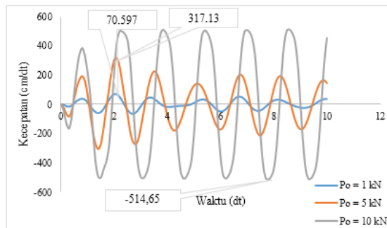
Gambar 8. Riwayat Waktu vs Kecepatan Dengan Variasi Nilai P_0 Akibat Beban Cosinus Pada Lantai Sepuluh
