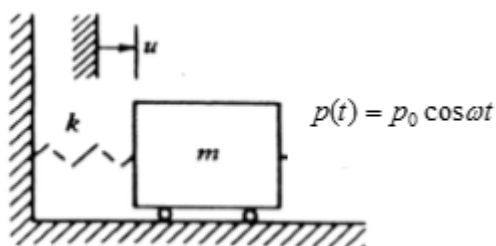
Gambar 3. Gerak Harmonik Dari Sistem SDOF Tak Teredam
